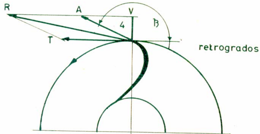
Figura 38. Álabes para ángulos de salida muy grandes.
