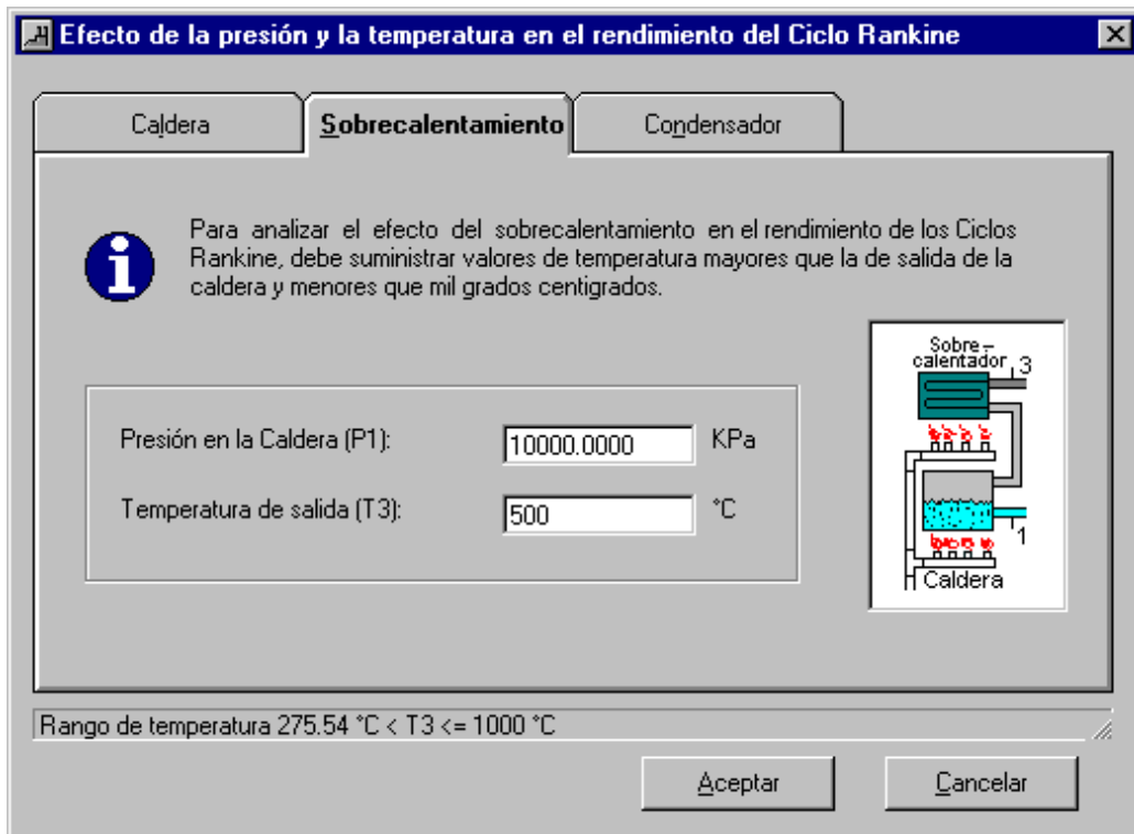
Figura 13. Efecto de la presión y la temperatura en el rendimiento del Ciclo Rankine
