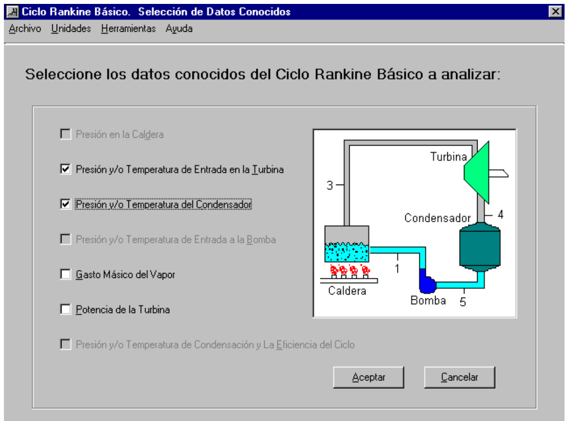
Figura 4. Selección de datos conocidos.
