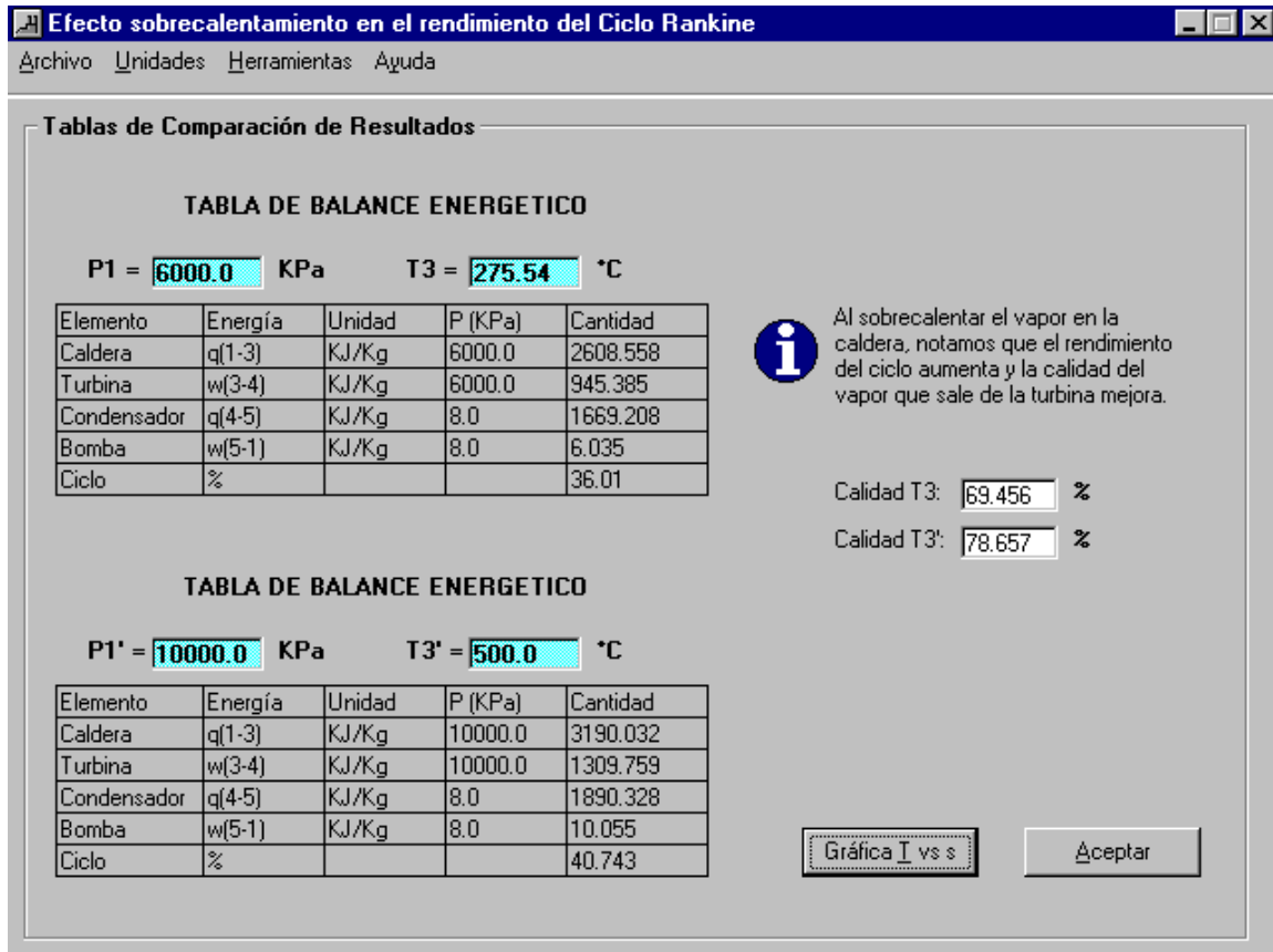
Figura 14. Soluciones. Efecto de la presión y la temperatura en el rendimiento del Ciclo Rankine
