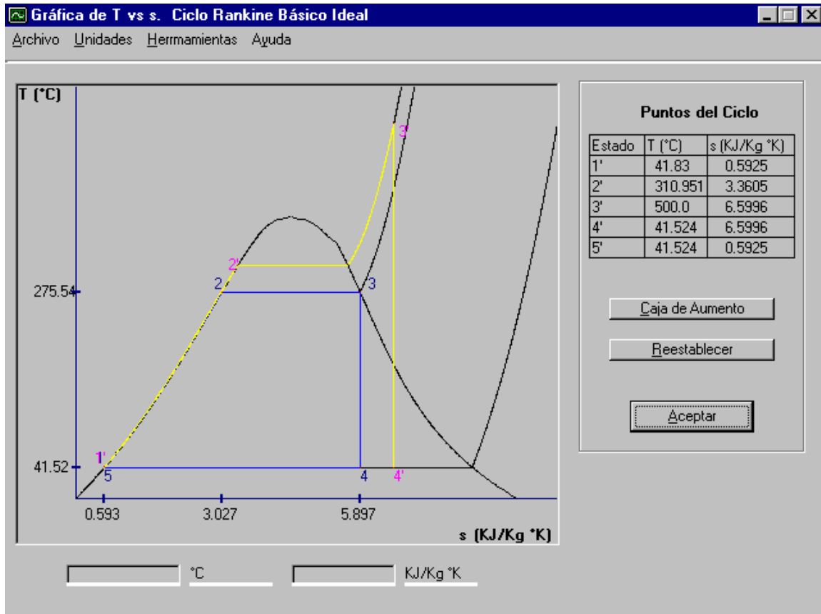
Figura 15. Gráfica T vs s. Efecto de la presión y la temperatura en el rendimiento del Ciclo Rankine
