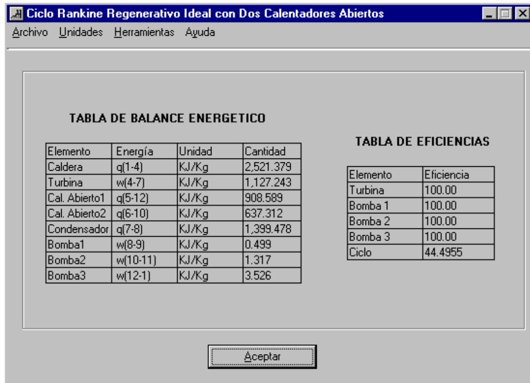
Figura 11. Soluciones, Ciclo Rankine Regenerativo.
