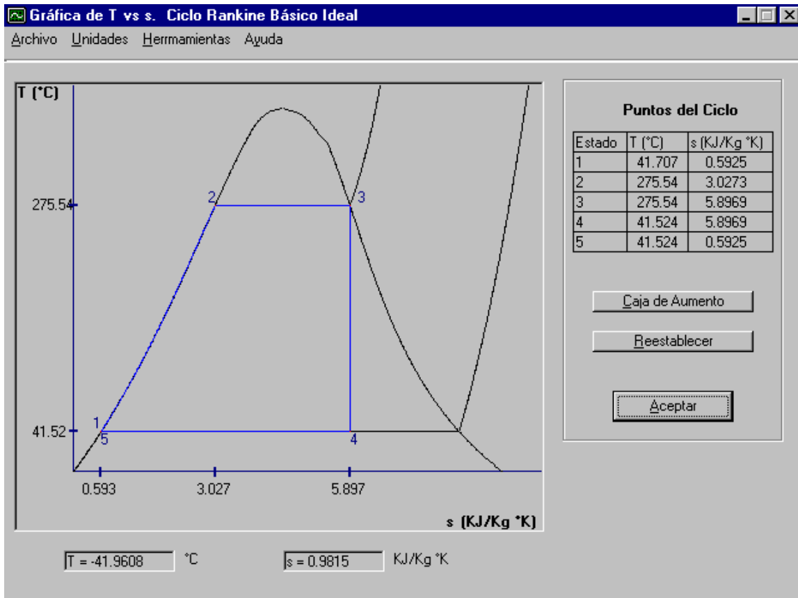
Figura 12. Pantalla de Gráfica T vs s.
